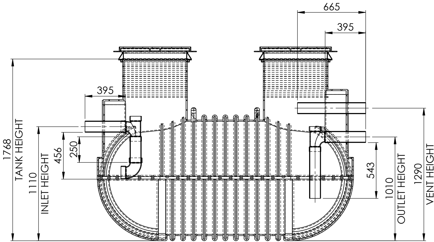
SECTION A-A
