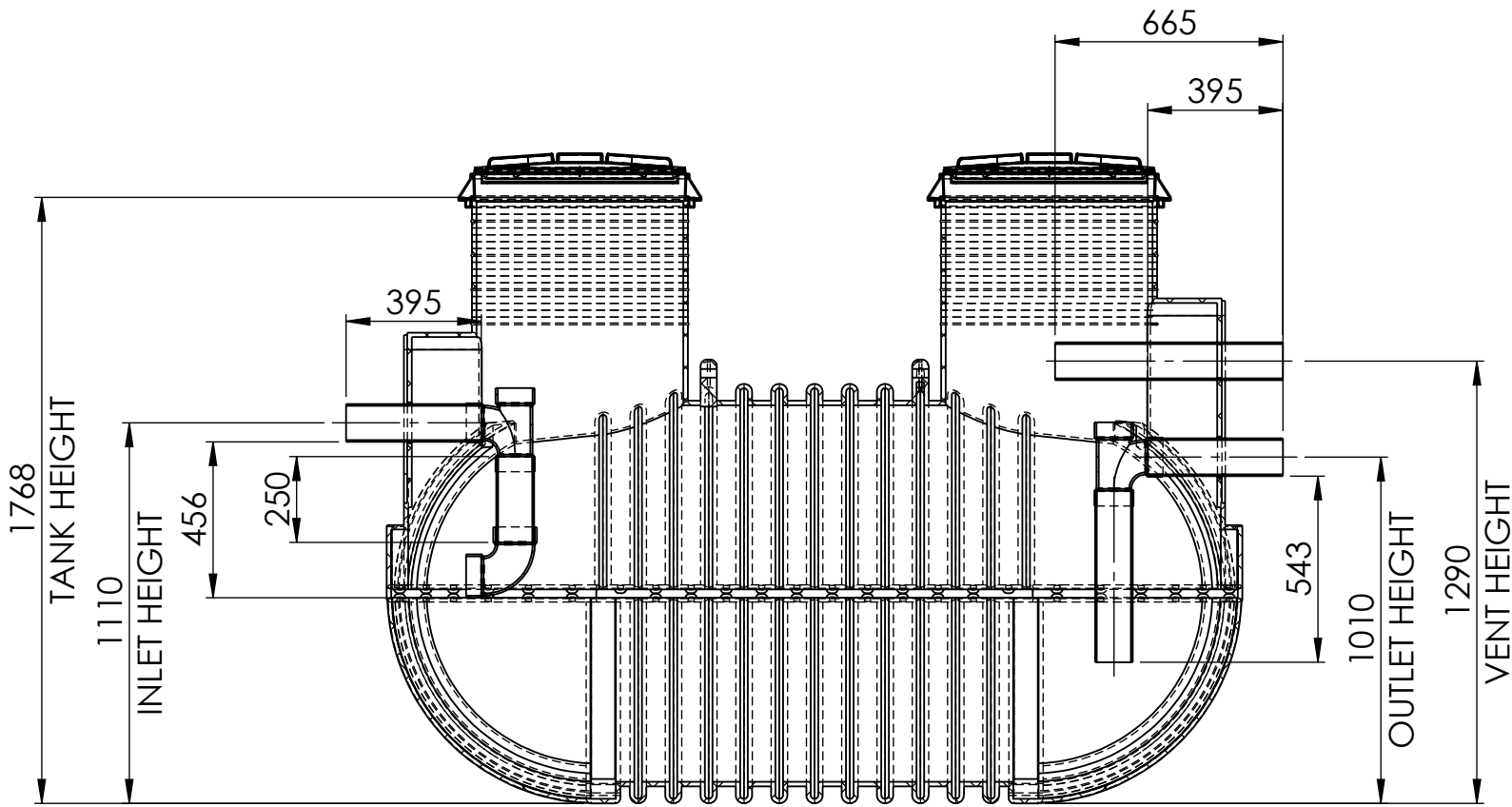
SECTION A-A
